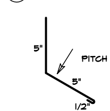
9 ENDWALL
