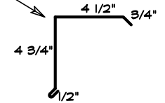
4b 2X4 MINI GABLE
